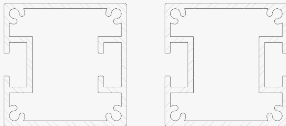
Dwarsdoorsnede
