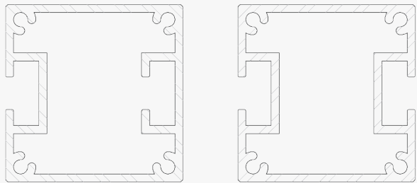
Dwarsdoorsnede
