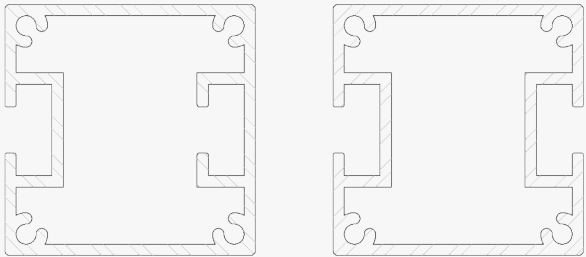
Dwarsdoorsnede
