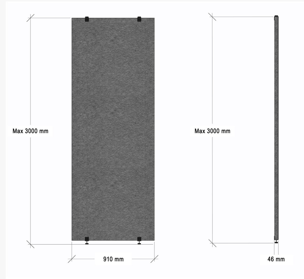
Maatvoering
