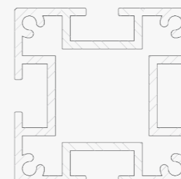
Dwarsdoorsnede
