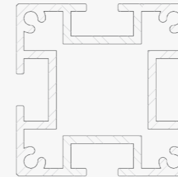
Dwarsdoorsnede
